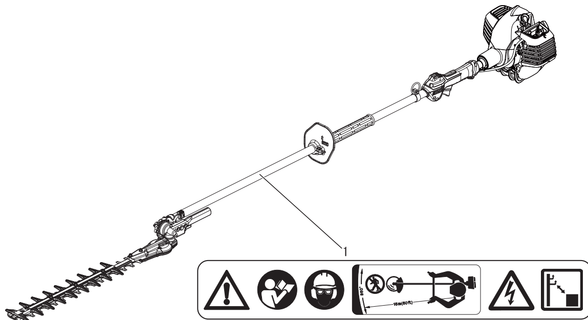
1. Varningsdekal (artikelnummer 890617-12361)
