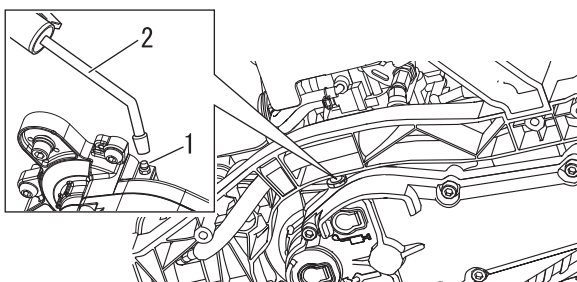
1. Smörjnippel
