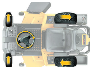
SYNCHRO-STEER-TEKNIK
